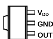
SOT-89
