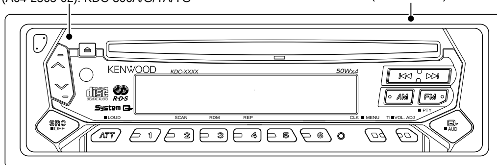
Escutcheon (B07-3054-02)
