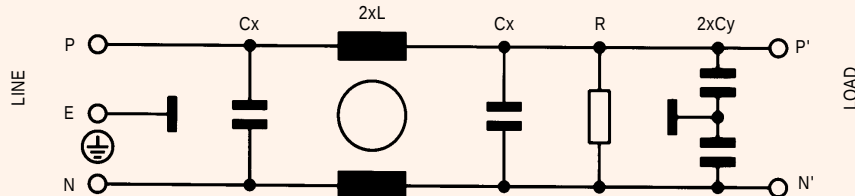
FN 9675 (16A)
