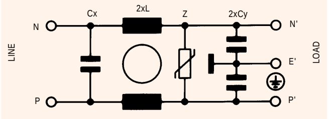
FN 332Z
