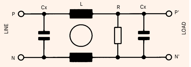
FN 402B
