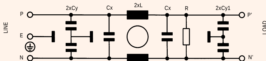
FN 9676 (16A)
