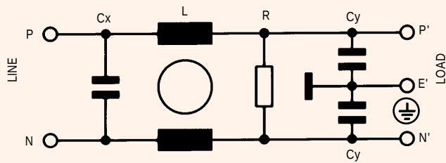
FN 402
