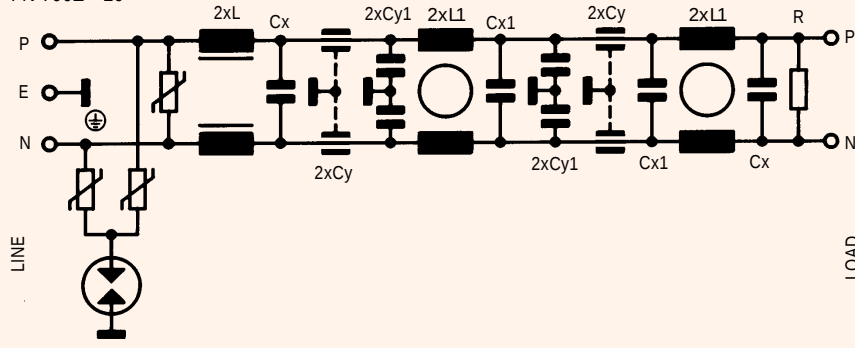
FN 700Z - 20
