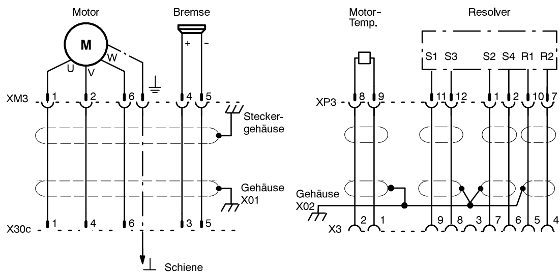
Abb. 8 Leitungsplan Antrieb A3
