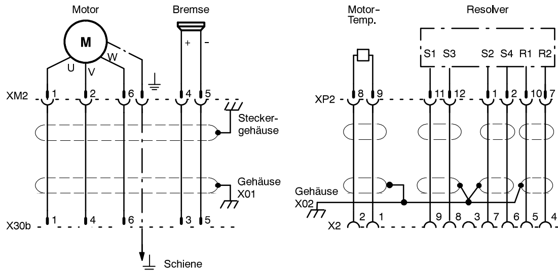
Abb. 7 Leitungsplan Antrieb A2
