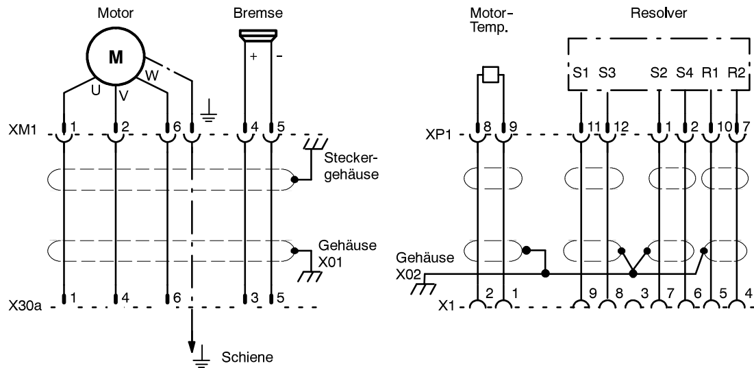
Abb. 6 Leitungsplan Antrieb A1
