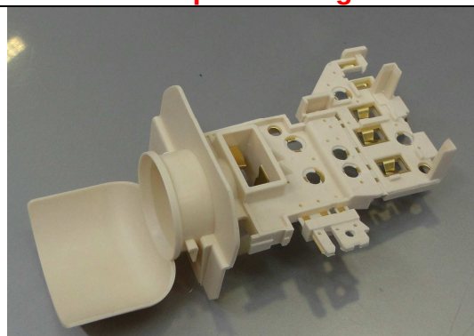
Detailansicht: neue Konfiguration Lampenfassung
