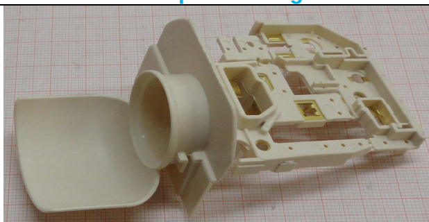
Detailansicht: alte Konfiguration Lampenfassung
